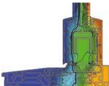
Isotermenvverloop Corona CT70 HS Tracé des isothermes Corona CT 70 HS
